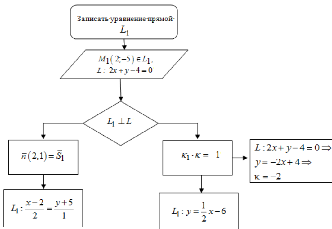
Рис. 3. Графическая схема-алгоритма
