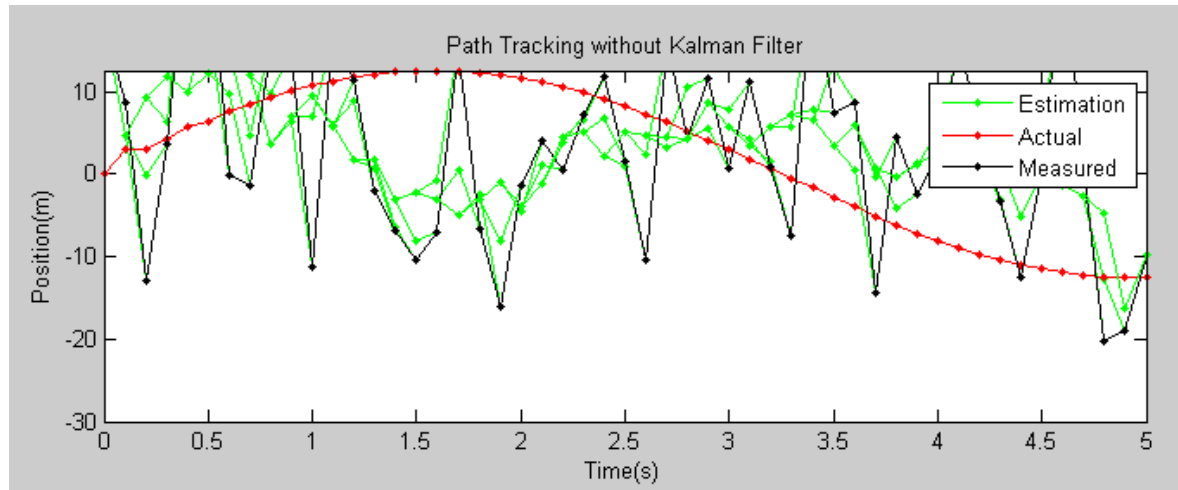
Рис. 2 – Результаты моделирования сопровождения кусков руды без фильтра Калмана
