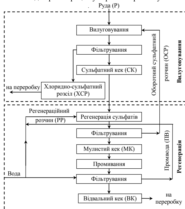
Рис. 1. Принципова схема сульфатного вилуговування
