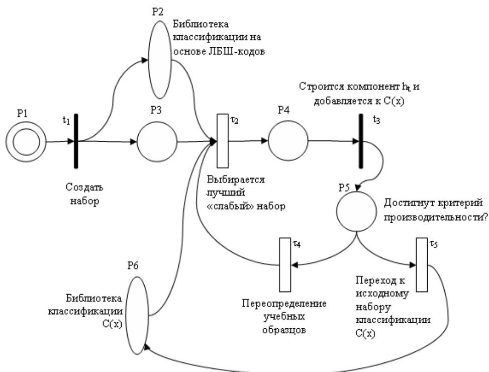
Рис. 2. Алгоритм распознавания
