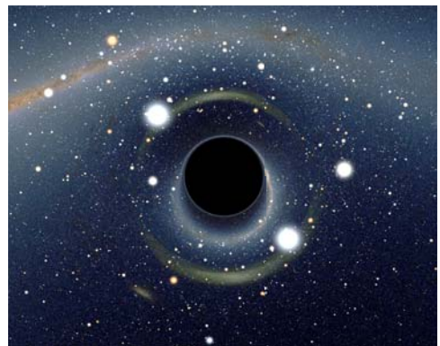
Гравітаційні викривлення, спричинені чорною дірою перед Великою Магелановою Хмарою (художнє зображення із вікіпедії)
