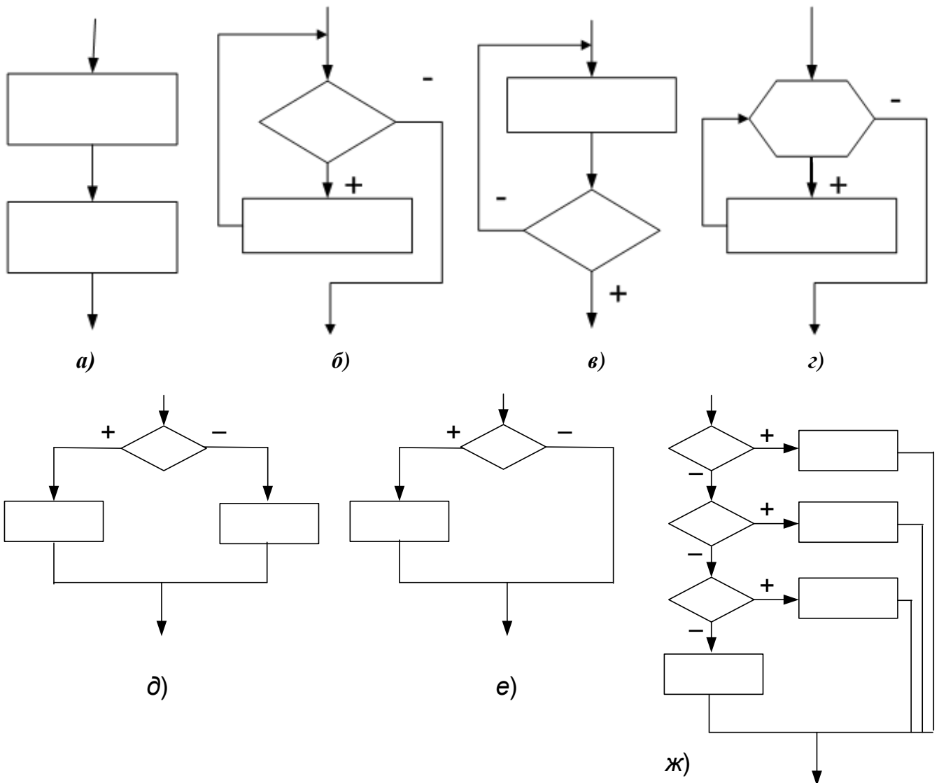
Рис. 4. Основні алгоритмічні конструкції, представлені блок-схемами: а – лінійна ділянка алгоритму, б – цикл з передумовою, в – цикл з посту мовою, г – цикл з параметром, д - розгалуження (повна форма), е - розгалуження (неповна форма) [17].
