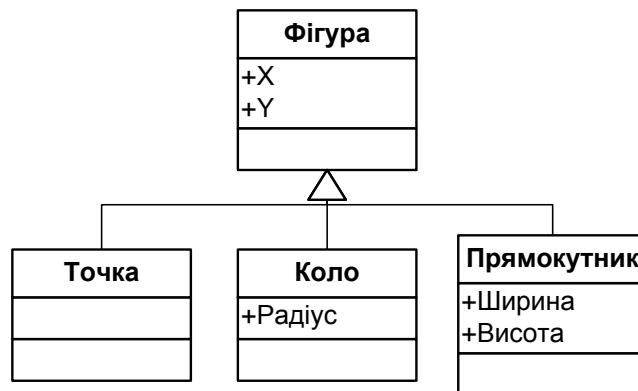
Рис. 6. Приклад спадкування.
