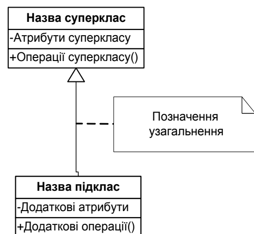
Рис. 5. Узагальнення.
